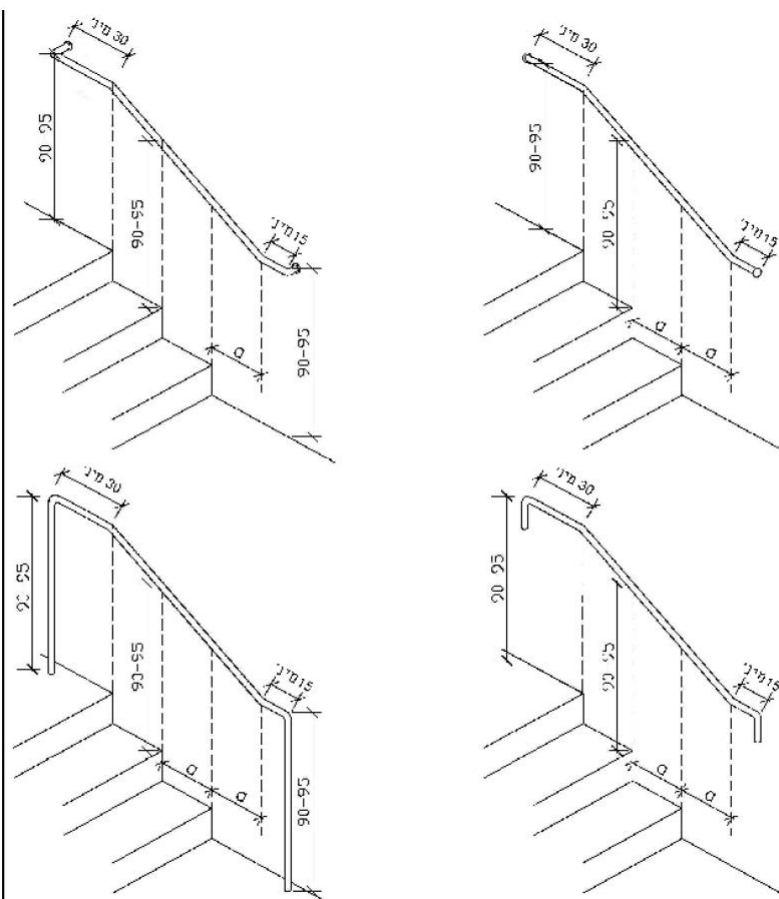
ציור 10 – דוגמות לקצות בתי-אחיזה למדרגות (המידות בסנטימטרים)
