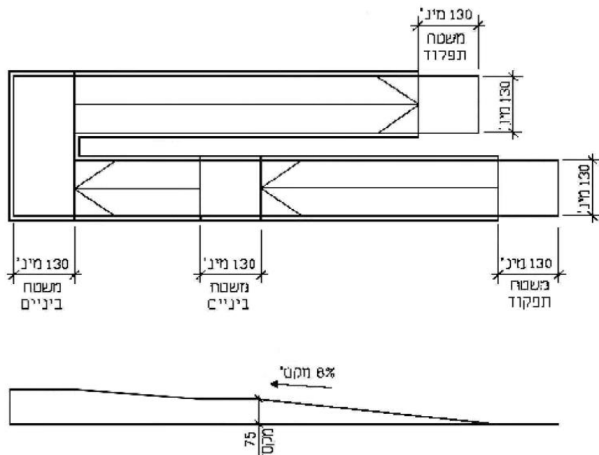
ציור 2 – משטחי ביניים בכבש (המידות בסנטימטרים)
