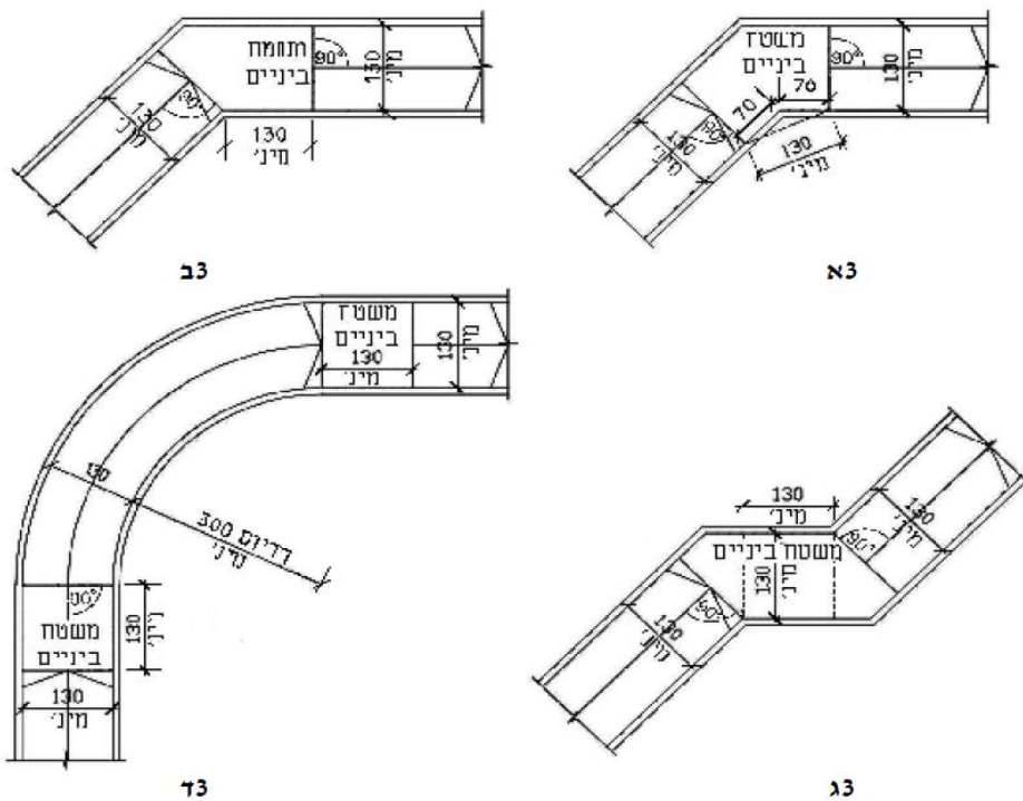
ציור 3 – דוגמות למפגש בין כבש למשטח ביניים (המידות בסנטימטרים)
